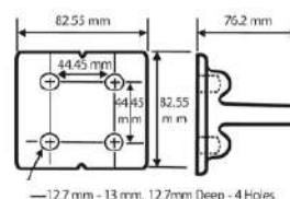
Fig. B : HCCP - 4120 / HCCP - 4240
